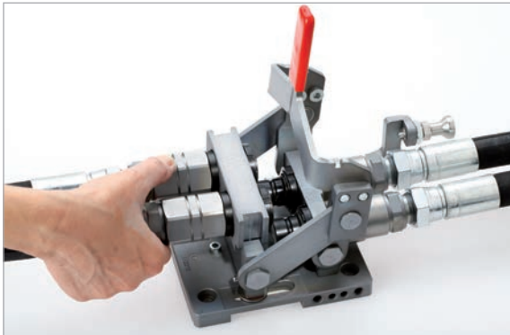
Wechselplatte in das System einstecken
